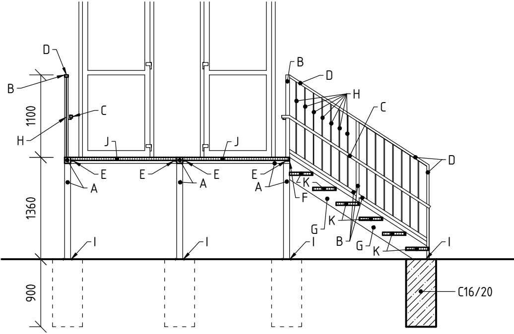
ŘEZ A-A'
