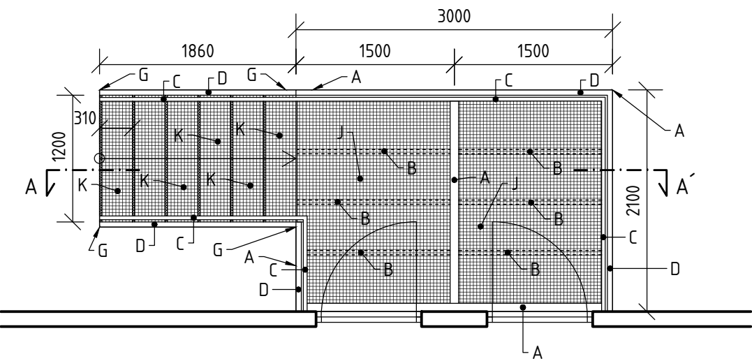
PŮDORYS
