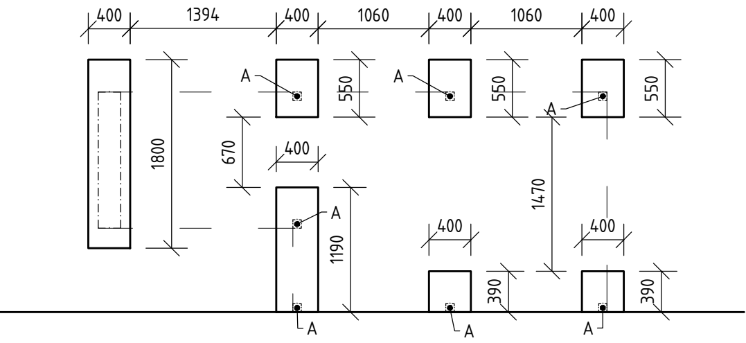
ZÁKLADY
