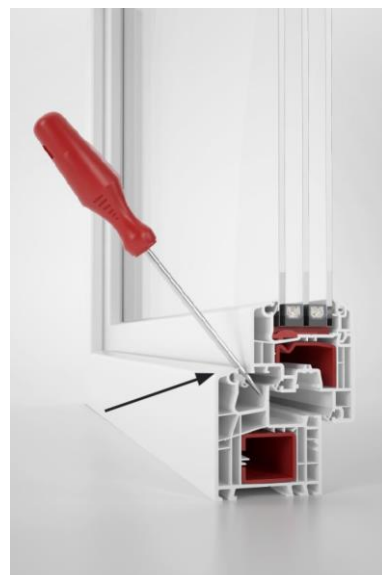
Pevná nalehávka - ochrana proti vniknutí
