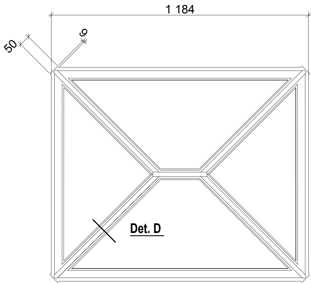
Půdorysný pohled
